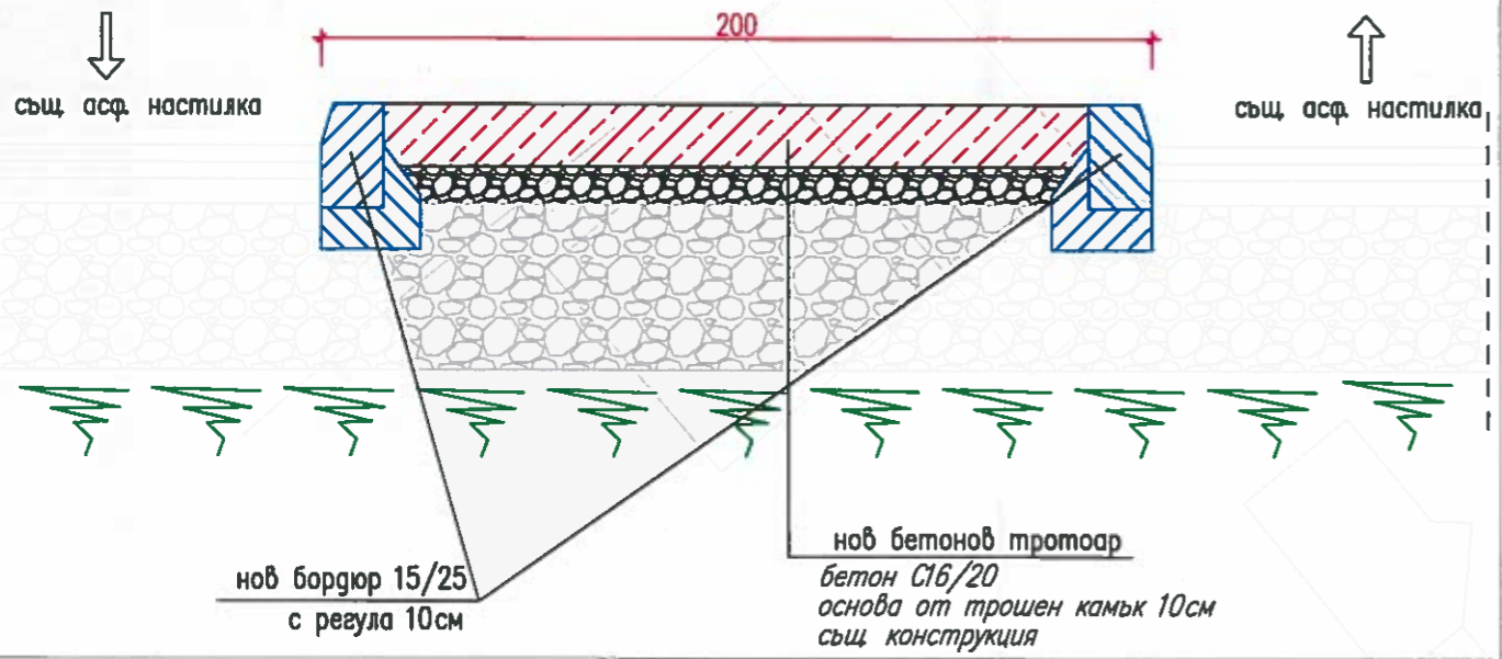
детайл при обособяване на централен остров от бетонов тротоар в оста на уличното платно М 1:20
